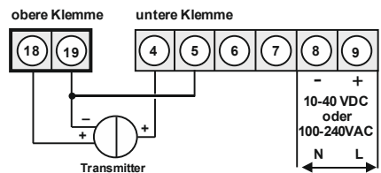
3-Leiter-Sensor 0-20 mA
