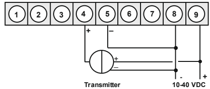
M3 in Verbindung mit einem 3-Leiter-Sensor 0/4-20 mA
