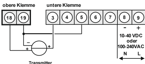
3-Leiter-Sensor 0-10 V
