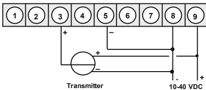
M3 in Verbindung mit einem 3-Leiter-Sensor 0-10 V
