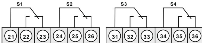
Relais 1 und 2
