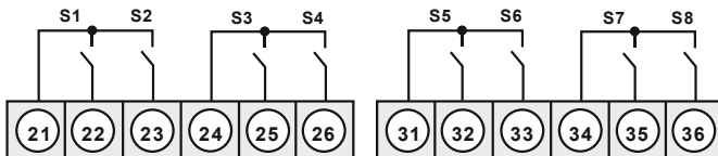
8 PhotoMos-Ausgänge
