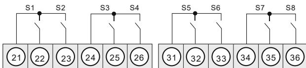
8 PhotoMos-Ausgänge
