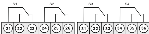
Relais 1 und 2
