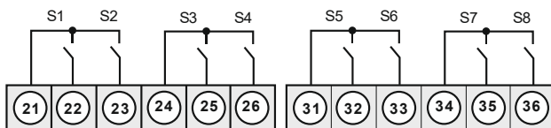
8 PhotoMos-Ausgänge
