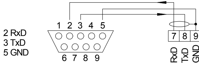
Anschlussbeispiel an die serielle Schnittstelle eines PC an ein GxB Gerät
