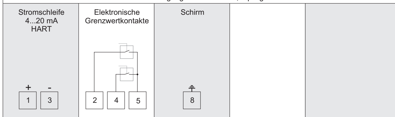
Belegung Stecker M12x1, 8-polig
