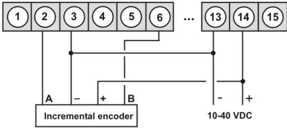
Incremental encoder
